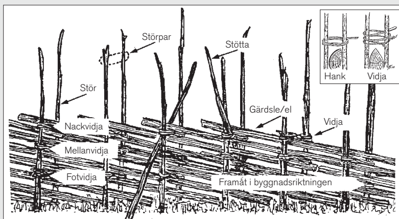
FIGUR 3. | Hankgårdsgårdens uppbyggnad (efter Hagander, 1995). Den infällda bilden visar att hanken är ringformig och träs över störrparet, medan vidjan binds som en åtta runt störrarna (efter ULMA:s frågelista nr 15 Hägnader. SOFI).
