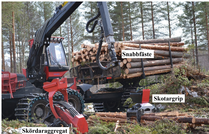
Figur 5. Konzeptdrivaren Komatsu X19 med snabbfäste, här i samband med skifte mellan skördaraggregat och skotargrip. Skotargripen underlättar lossning, och skördaraggregatet möjliggör avverkning. Drivaren är ett exempel på ett enmaskinsystem som kan vara lämpligt för hyggesfritt skogsbruk. Foto: Rikard Lundqvist.
