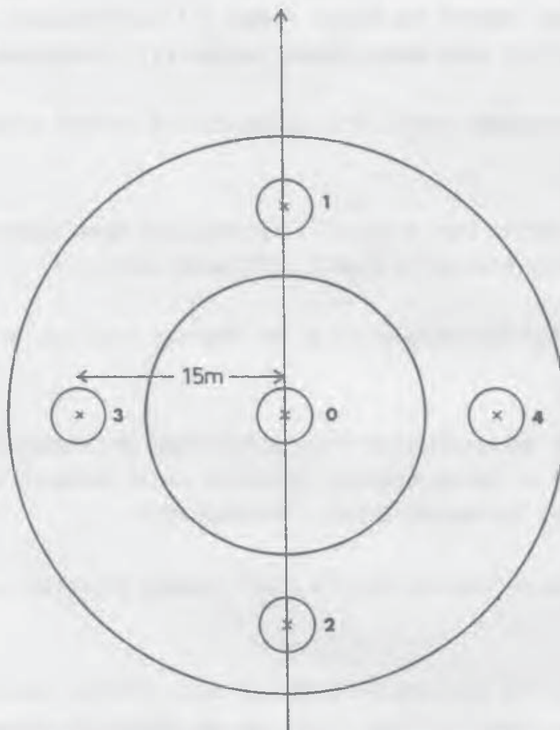
Planträkningsytornas placering inom 20 m-ytan.
