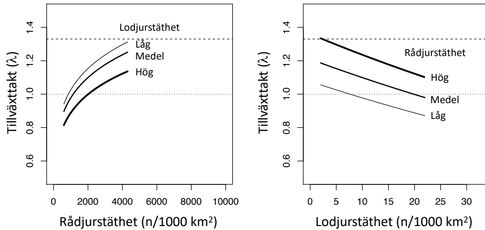
Figur 3. Den potentiella tillväxttakten utan legal jakt för lodjurspopulationen i mellersta och södra RFO i relation till rådjurstäthet (till vänster) och lodjurstäthet (till höger). Den nedre punktade linjen visar en potentiell tillväxttakt ( \lambda ) = 1 och den övre streckade linjen visar en potentiell tillväxttakt ( \lambda ) = 1,33, vilket ungefär visar på maximal potentiell tillväxttakt hos lodjur (Andrén m.fl. 2006). Till vänster visas olika tätheter av lodjur; låg = 5, medel = 10, hög = 20 lodjur/1000 km 2 . Till höger visas olika tätheter av rådjur; låg = 1000, medel = 2000, hög = 4000 rådjur/1000 km 2 . Från Andrén & Liberg (accepterat manuskript).
